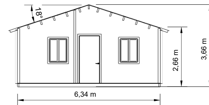
Sektion
