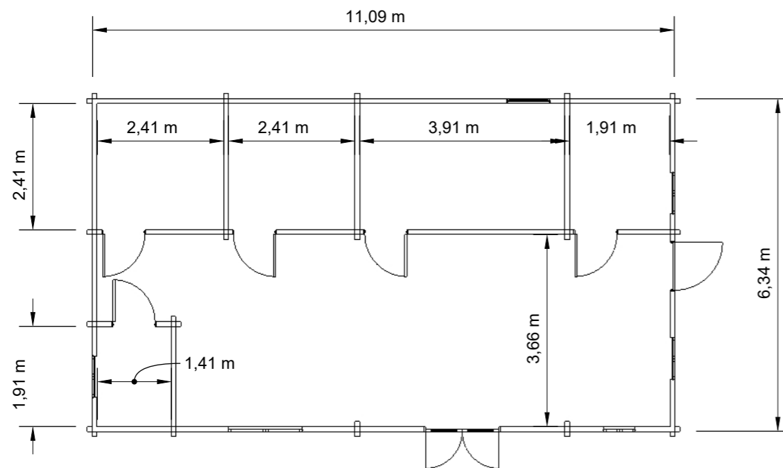
Planritning
