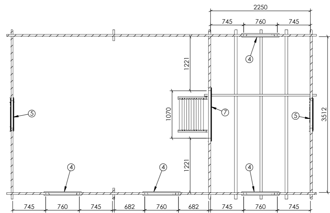
Plan loft
