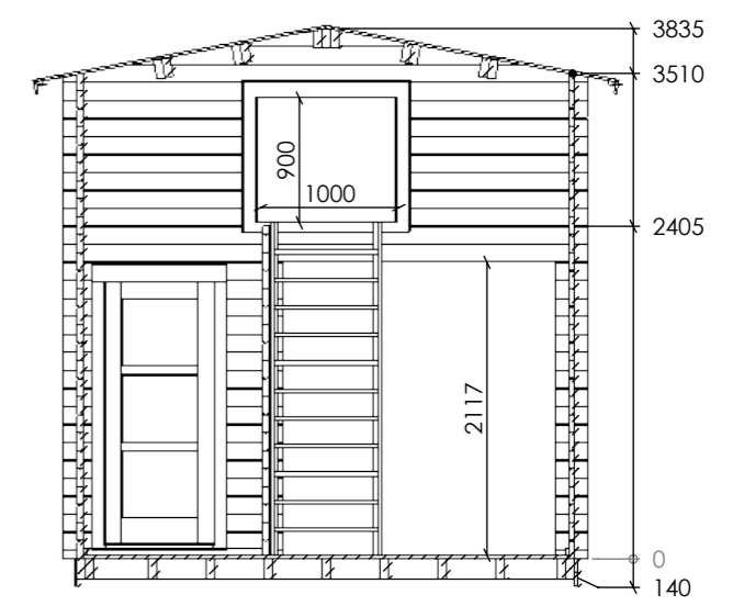
D-D
