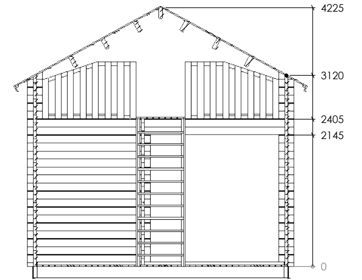
B-B
