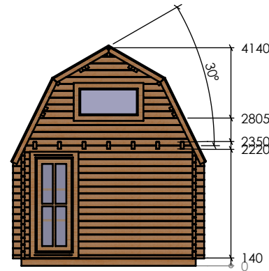
Facade A-B M1:100
