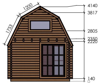
Facade B-A M1:100
